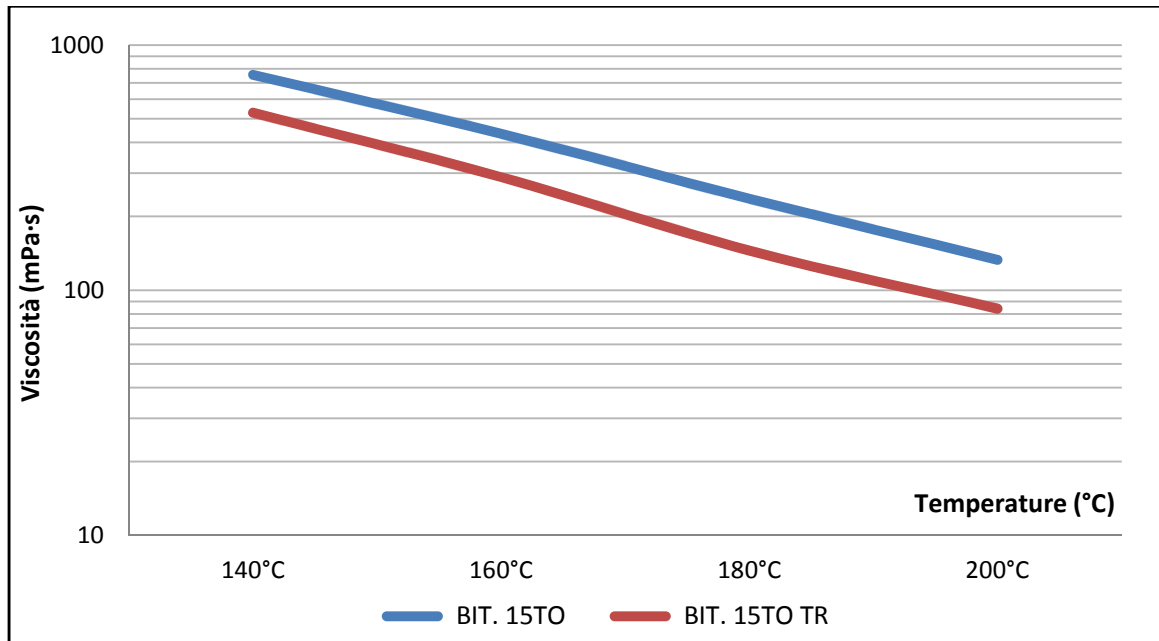
VISCOSITÀ DEL BITUME MODIFICATO BIT. 15 TR IN FUNZIONE DELLA TEMPERATURA (Curva di viscosità dinamica tipica)
